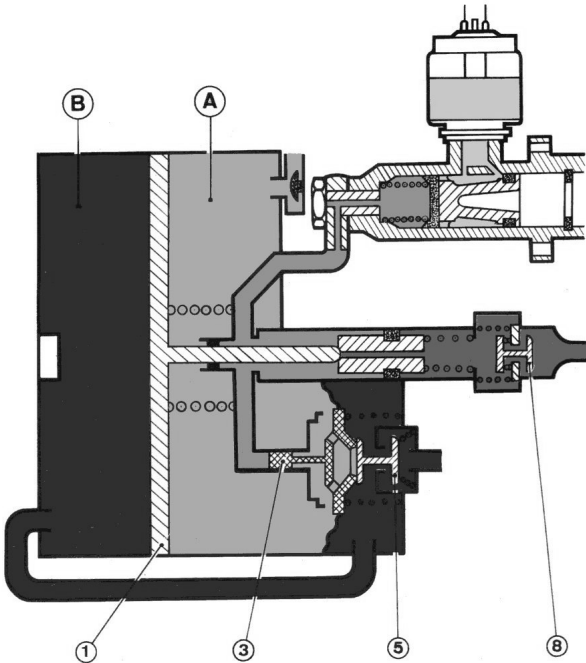
fig. 5 Position de freinage Maxi
