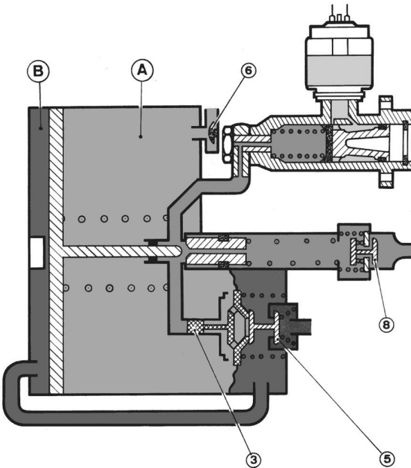
fig. 2 Début du freinage
